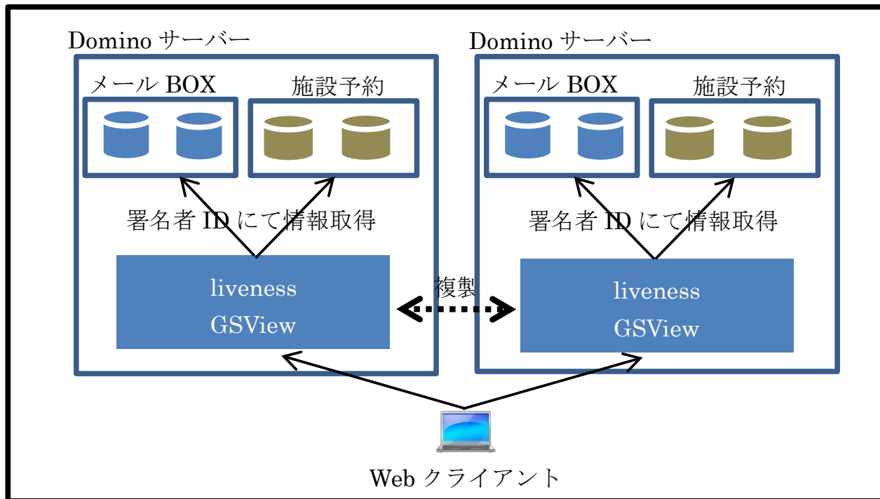
liveness GSView 概要図
